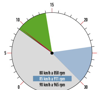
Caja de Cambios Scania G33CM velocidad OD
