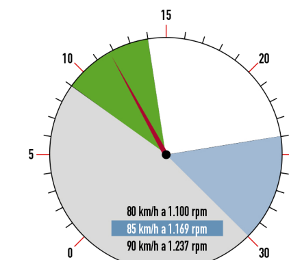
Caja de Cambios Scania G33CM velocidad 12°
